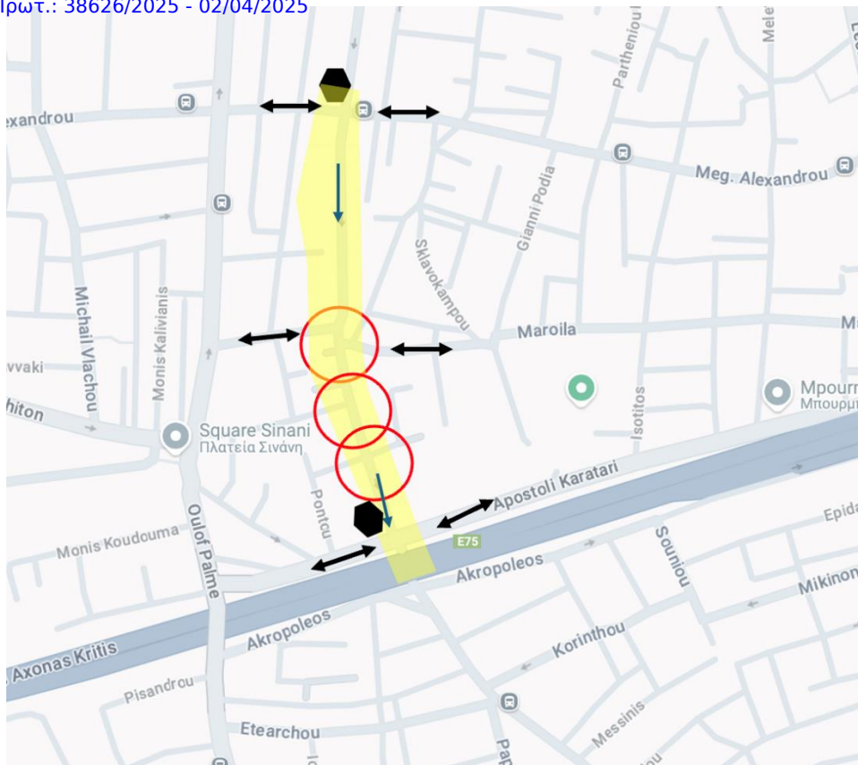
Εικόνα 4. κατευθύνσεις οδών, υφιστάμενη σήμανση P-2 και εντοπισμός ελλείψεων εντός περιοχής μελέτης Ακολουθούν φωτογραφίες σε διάφορες οδούς της περιοχής.
