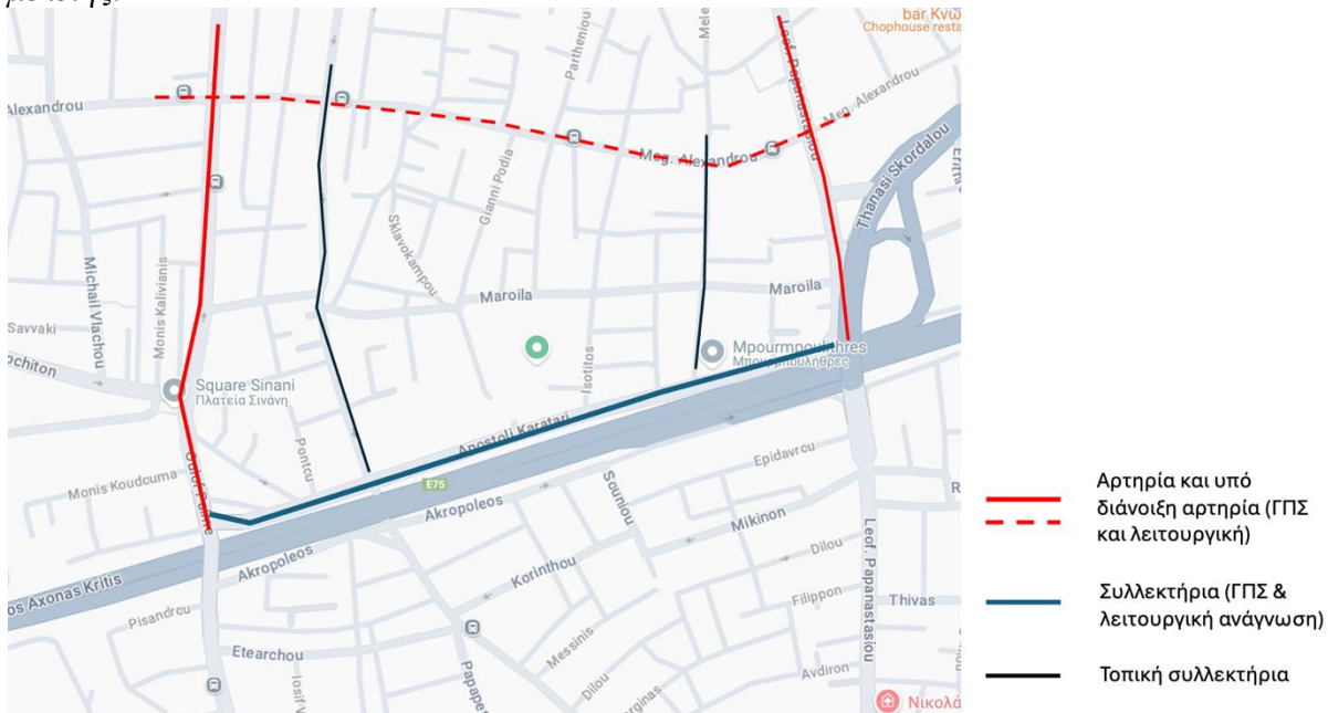
Εικόνα 3. λειτουργική ιεράρχηση στην περιοχή μελέτης
