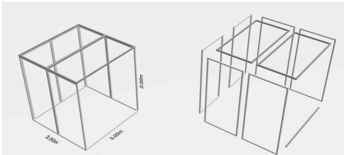
Μεταλλική κατασκευή 5
