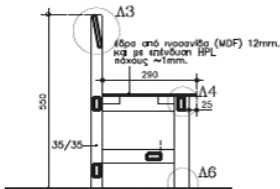
ΤΟΜΗ Τ1-Τ1 1:10
