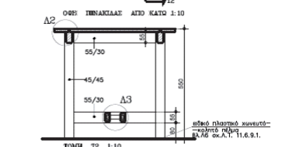
ΤΟΜΗ Τ2 1:10
