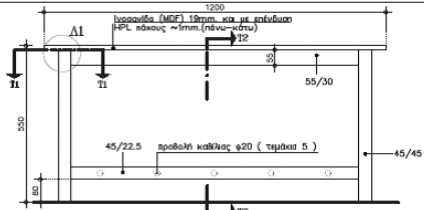
ΠΡΟΣΩΦΗ 1:10
