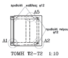
ΤΟΜΗ Τ2-Τ2 1:10
