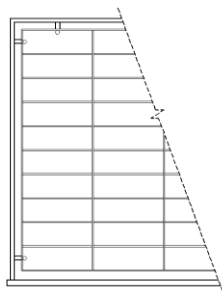
ΣΙΔΕΡΙΑ ΤΥΠΟΥ Σ1 Πλαίσιο και κατακόρυφες λάμες 40/6 Οριζόντια, σίδηρος κατασκευών Φ12 (διαπερνά τις κατακόρυφες λάμες 40/6)
