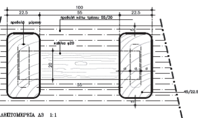
ΛΕΠΤΟΜΕΡΕΙΑ Δ3 1:1
