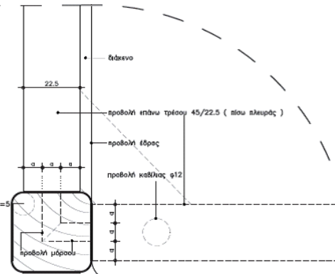
ΛΕΠΤΟΜΕΡΕΙΑ Δ1 1:1
