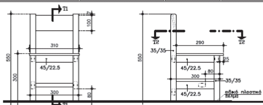
ΠΡΟΣΩΦΗ 1:10
