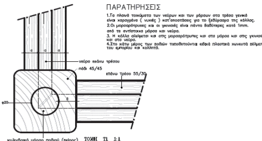
Κυλινδρικό μέρος ποδιού (πέρας) ΤΟΜΗ Τ1 1:1
