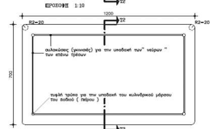
ΠΡΟΣΩΦΗ 1:10
