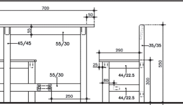
ΠΑΛΓΙΑ ΟΨΗ 1:10
