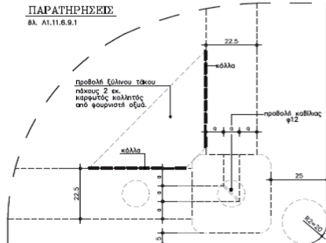
ΛΕΠΤΟΜΕΡΕΙΑ Δ2 1:1
