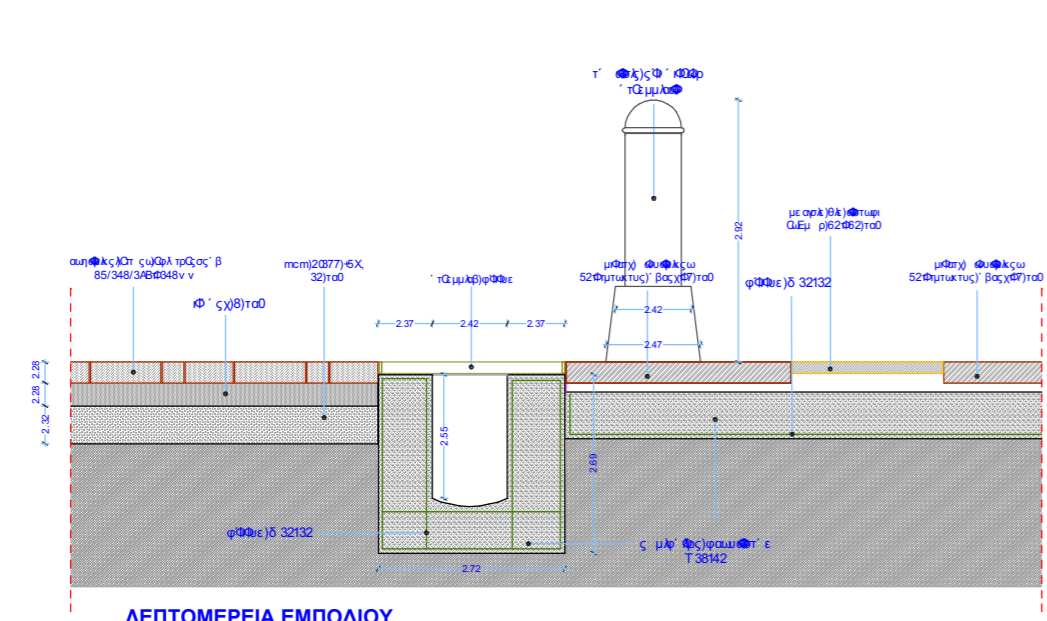
ΛΕΠΤΟΜΕΡΕΙΑ ΕΜΠΟΔΙΟΥ ΑΥΤΟΚΙΝΗΤΩΝ ΚΛΙΜΑΚΑ 1/20
