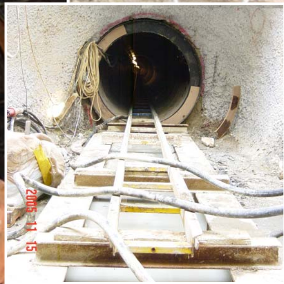
Κεντρικός συλλεκτής ακαθάρτων – όμβριων περιοχής Μεσσαμπελιών
