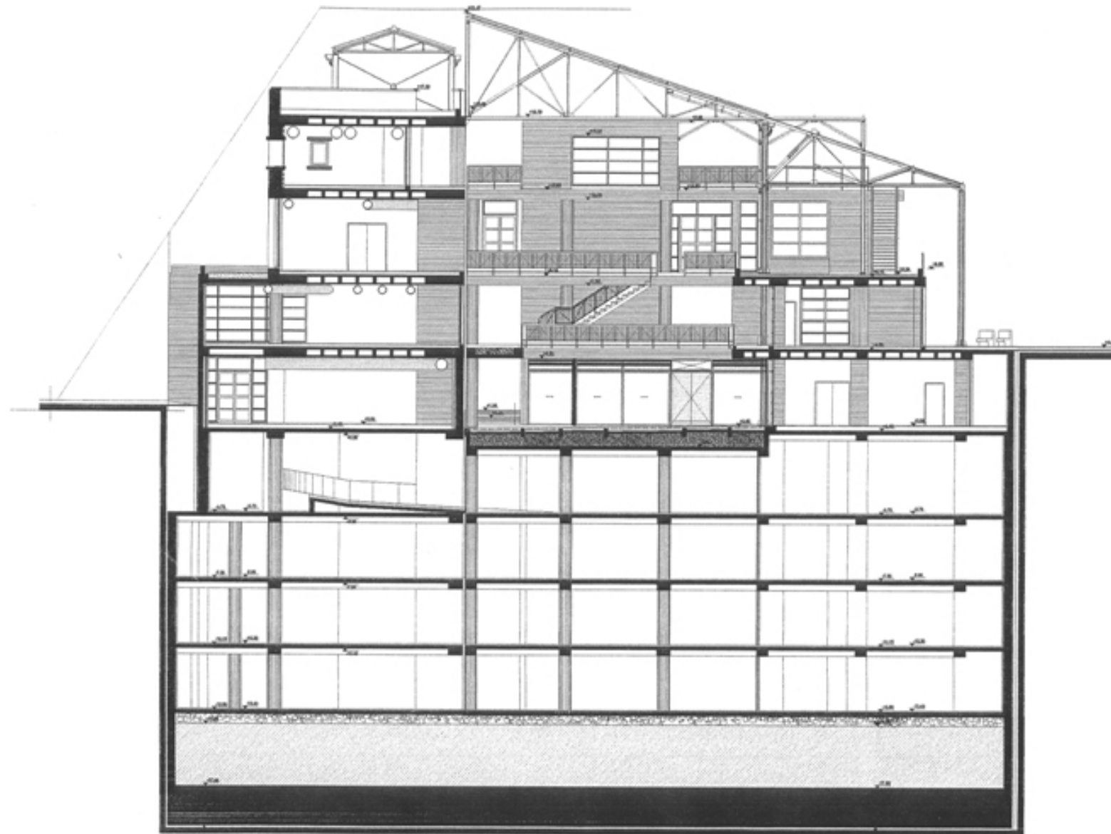
ΤΟΜΗ Β-Β 1:250
